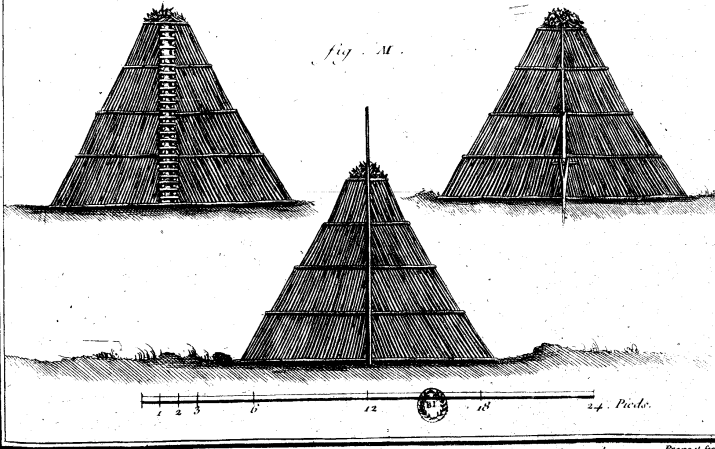
Œconomie Rustique; Charbon de Bois. Deffroy del.
